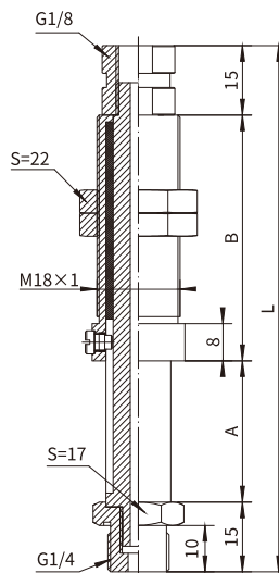
KI14 10-F-A18
